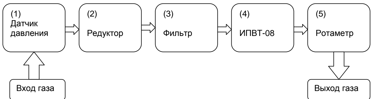
Рисунок 3.19 (а) Структурная схема системы пробоподготовки газов СПГ-Н
