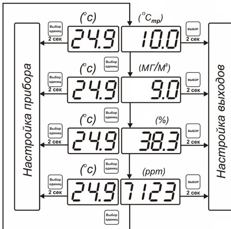
Рисунок 6.1 Режим РАБОТА
