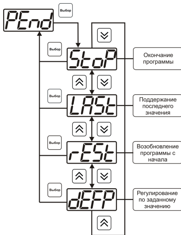
Рисунок 6.33 Меню настройки условий окончания программы
