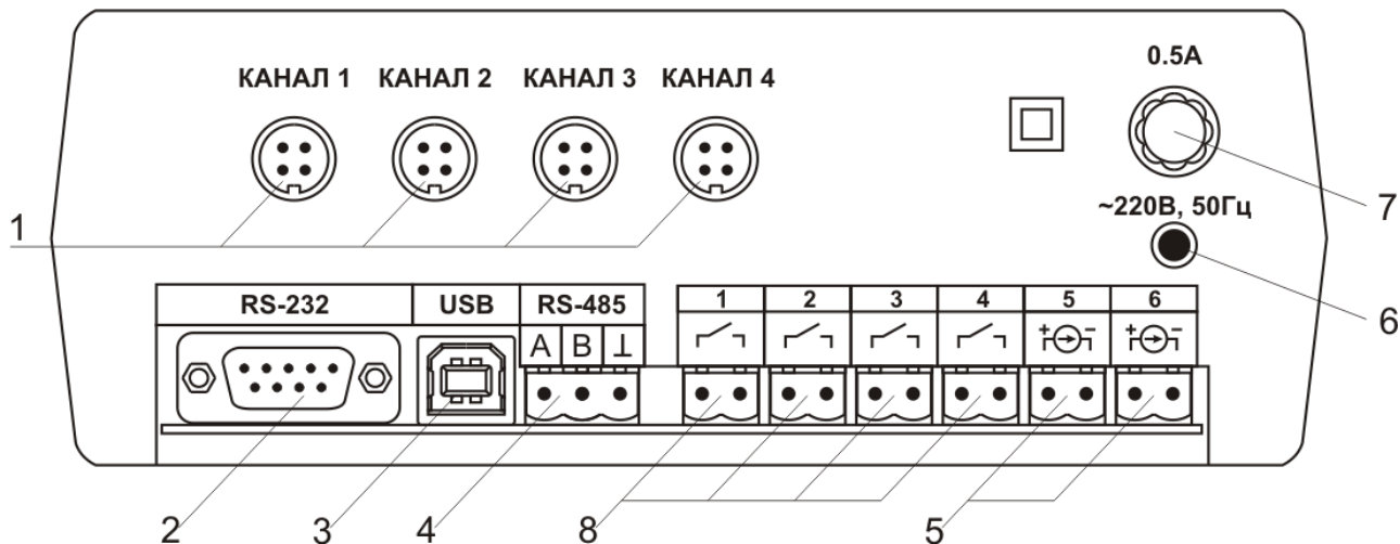
Рисунок 3.2 Задняя панель приборов ИВГ-1 /2-С, ИВГ-1 /4-С.
