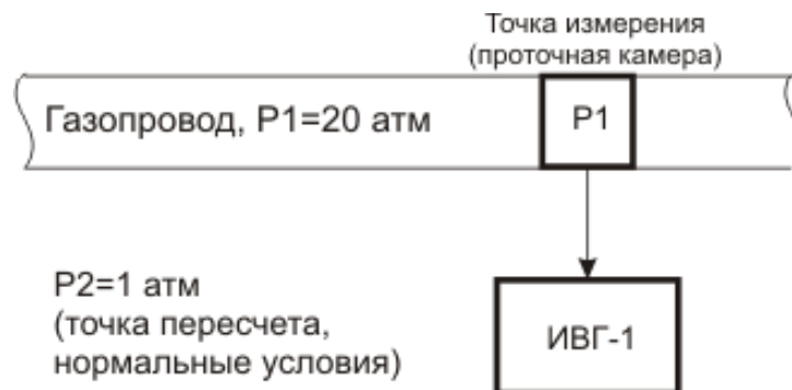
Рисунок 6.13 Пример использования пересчета показаний влажности.
